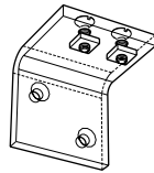
4140 (t.b.v. 4100) 5140 (t.b.v. 4200 & 5100) muurbeugel plexiglas 5 cm, t.b.v. NEN 1010
