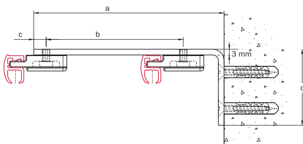
maten bij wandmontage met metalen afstandsteunen (zie tabel) en dekselsteunen 2150
